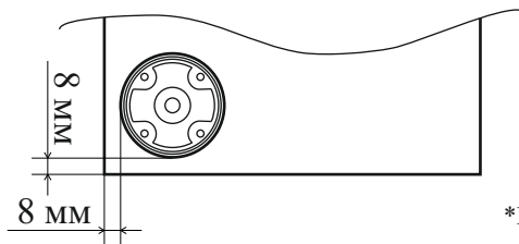
(рис.№4) СХЕМА ПРИСАДКИ ОПОР-НОГ
