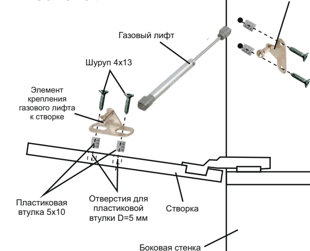
СХЕМА КРЕПЛЕНИЯ ГАЗОВОГО ЛИФТА
