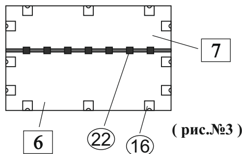
СХЕМА РАСПОЛОЖЕНИЯ ФИКСАТОРОВ
